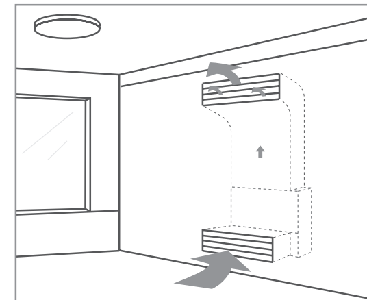
Пример установки канального блока в вертикальном положении.
