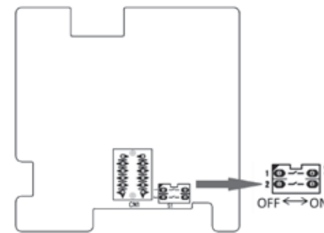
Рис. 28. Схема DIP-переключателей
